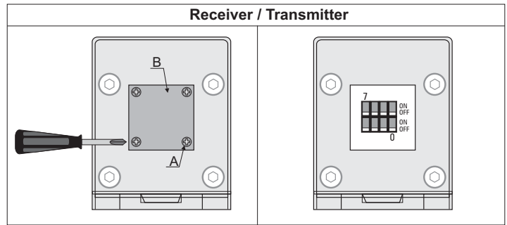
Fig. 1: Selettori - Switch
